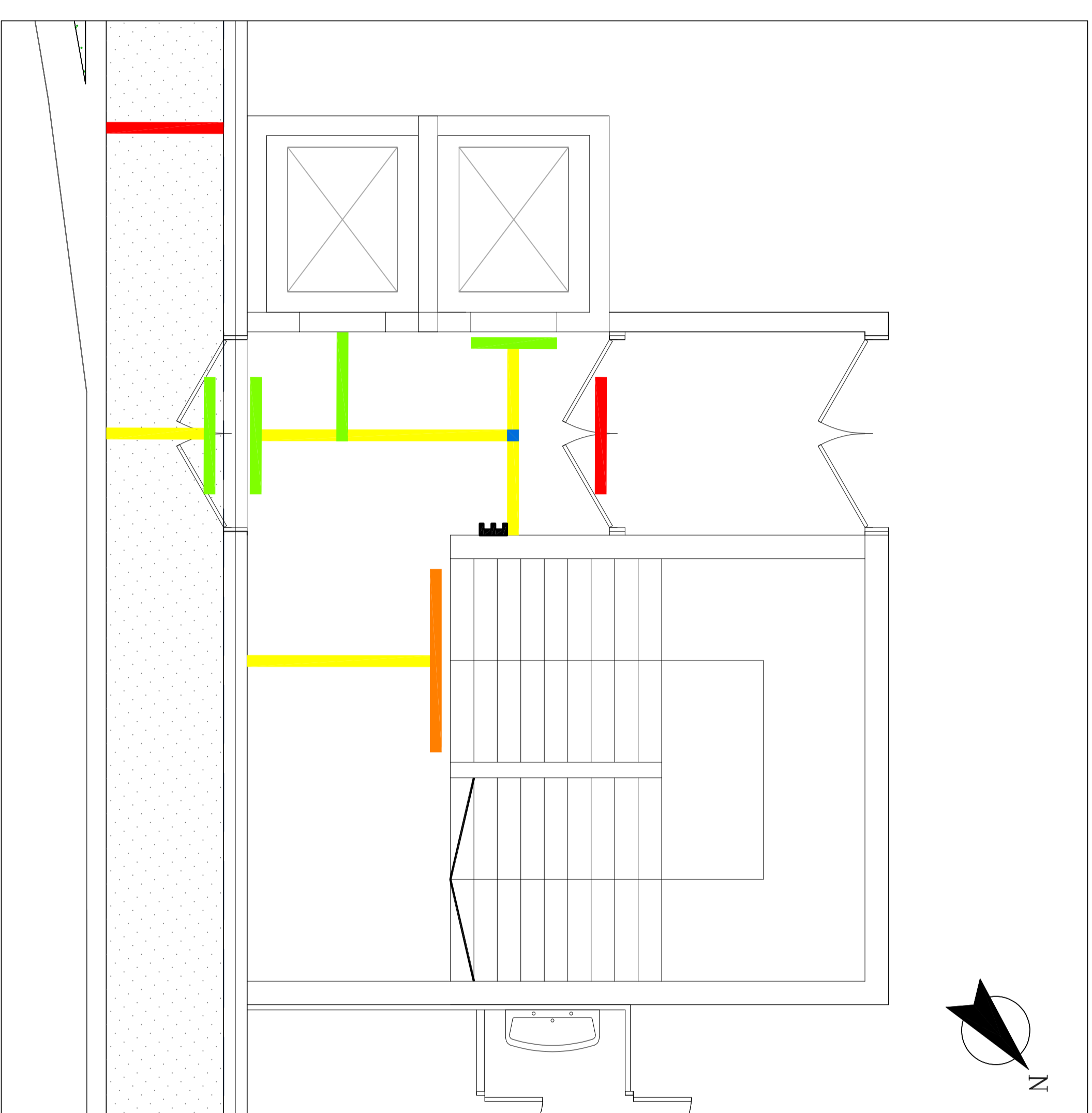
Particolare Ingresso Piano Terra scala 1:50
