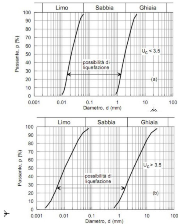
Figura 7.11.1 – Fusi granulometrici di terreni suscettibili di liquefazione.
