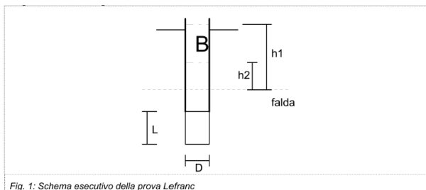
Fig. 1: Schema esecutivo della prova Lefranc
