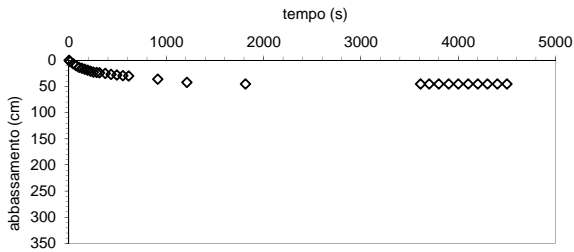
curva di svaso
